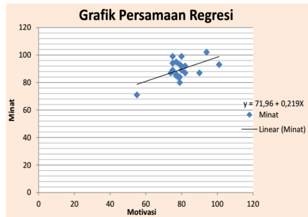
Gambar. 3 Grafik Persamaan Regresi
